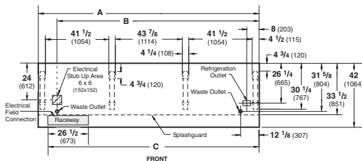
D5X-E, D5X-EP, D5X-LE, D5X-LEP, D5X-HE, D5X-HEP Plan View
